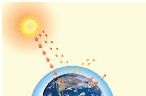
चित्र 13.2 — पृथ्वी पर हरितगृह प्रभाव का आरेख
